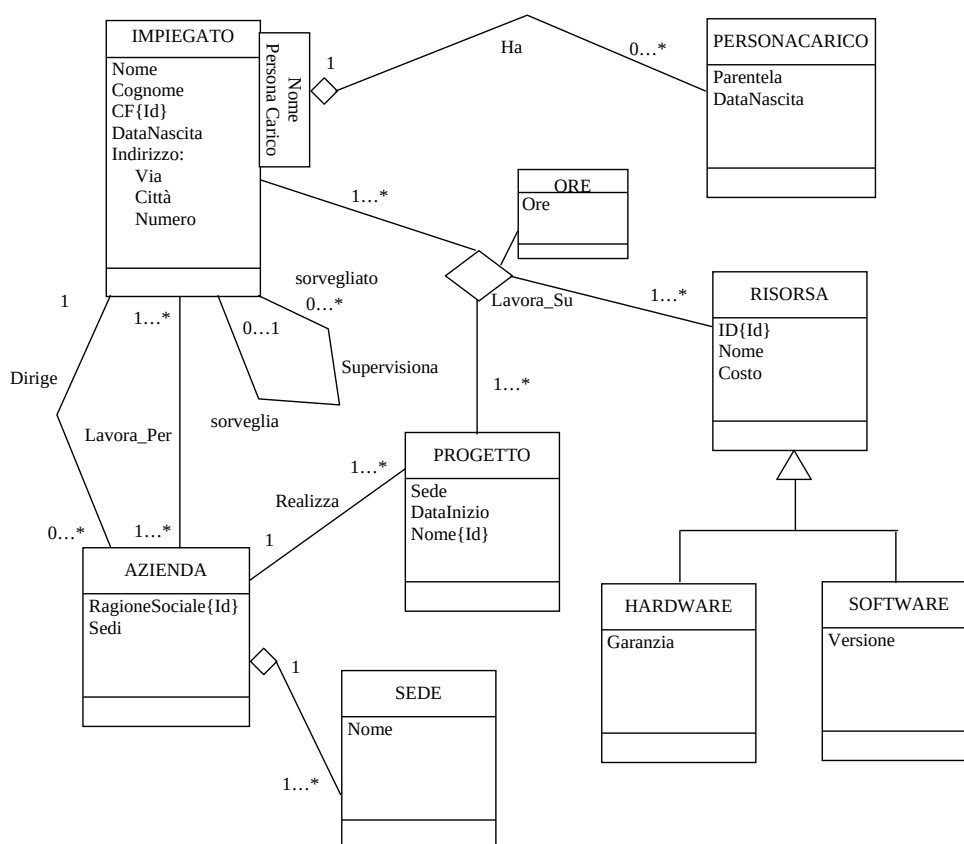
Figure 1: Il class diagram di un sistema per la gestione di una azienda
